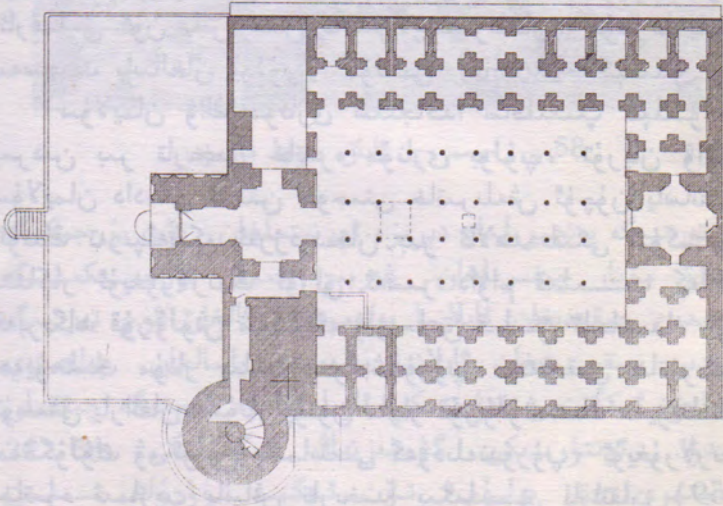
59 - رەسىم — سۇلايمان ۋاڭ مۇنارى
