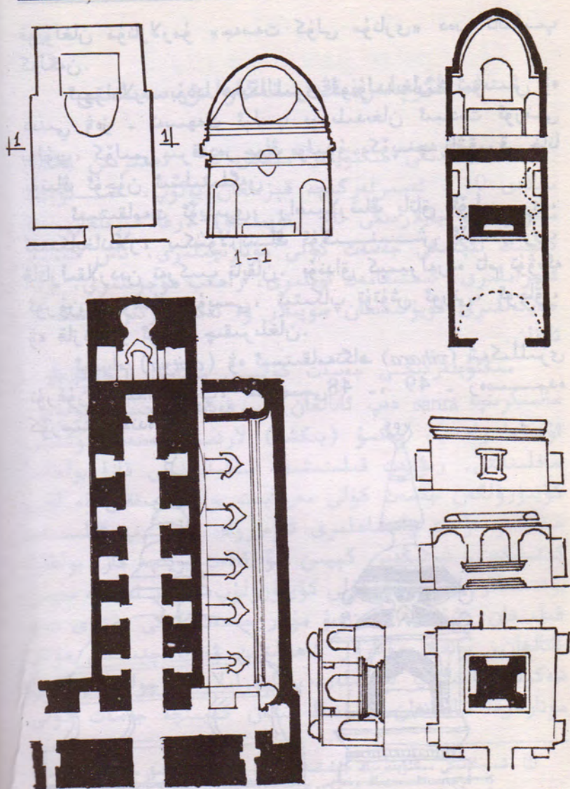
49 - رەسىم - شىنجاڭدىكى مىڭئۆيلەرنىڭ بىناكارلىق سىخىمىسى
