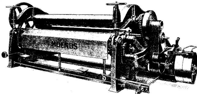
No. 334 Ausreck- und Abwelkmaschine „ESSORELLA“
